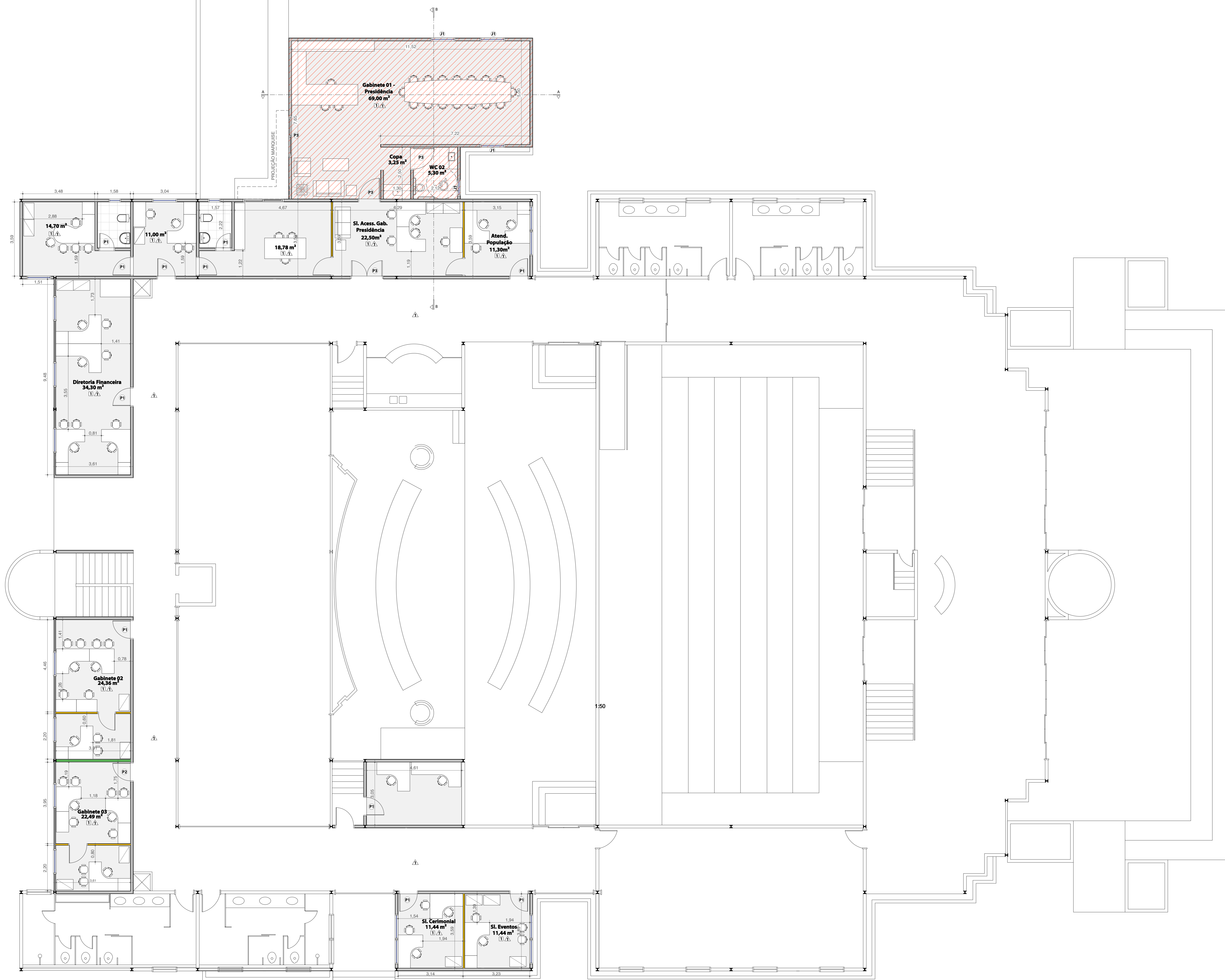
Planta Pavimento Térreo escala 1:75
